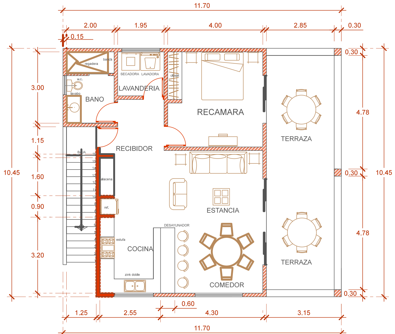
PLANTA ALTA VILLA 'C'
